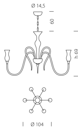
1022/10 CE 10 x MAX 42W E14
