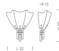
421/A1 CE 1 x MAX 42W E14
