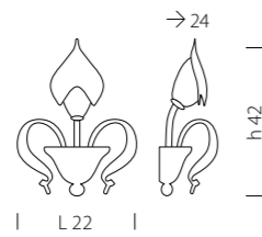
1479/A1 CE 1 x MAX 42W E14
