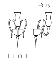
1022/A1 CE 1 x MAX 42W E14
