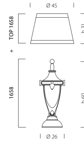
1658 + TOP 1658 CE 1 x MAX 42W E14 1 x MAX 70W E27
