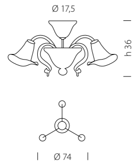
1480/3 CE 3 x MAX 42W E14
